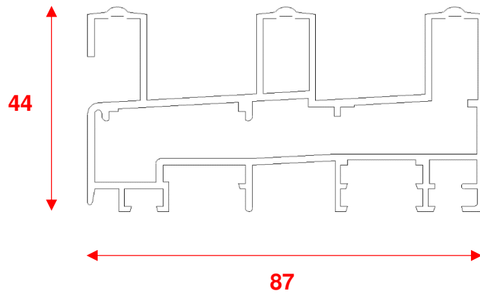
Telaio 3 binare (senza aletta battuta)
