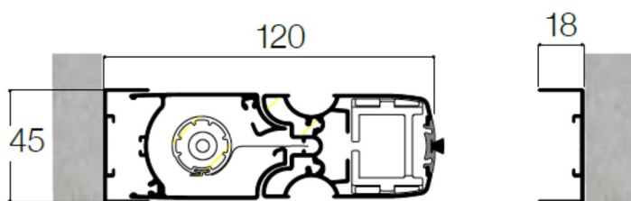
SEZIONE ORIZZONTALE
