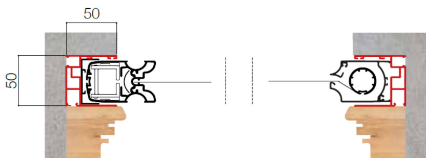
SEZIONE ORIZZONTALE INCASSO
