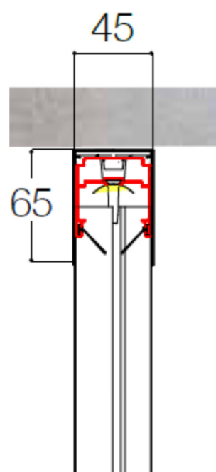
SEZIONE VERTICALE
