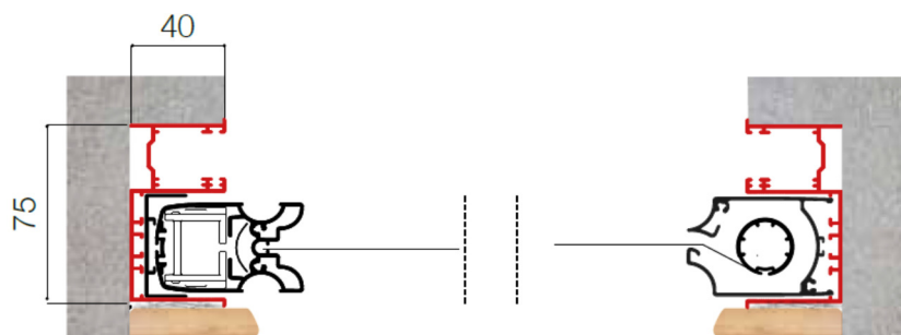
SEZIONE ORIZZONTALE INCASSO CON GUIDA TAPPARELLA
