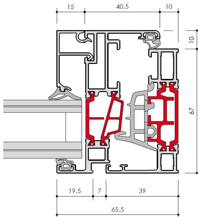
NODO TELAIO ANTA
