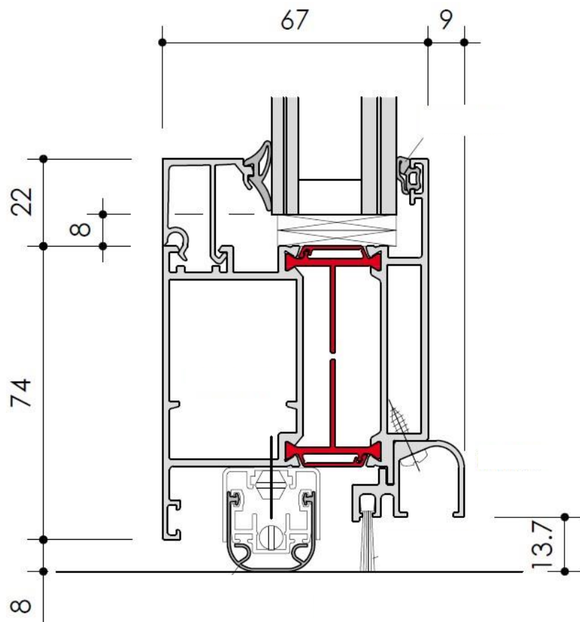
ZOCCOLO CON ANTA
